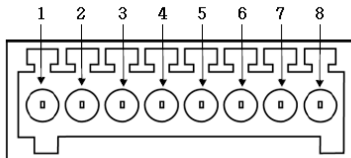
Рис.3.2. Схема клеммной колодки видеокамеры LTV-ICD*-423
