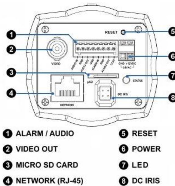
Рис.3.1. Задняя панель видеокамеры LTV-ICD*-423
