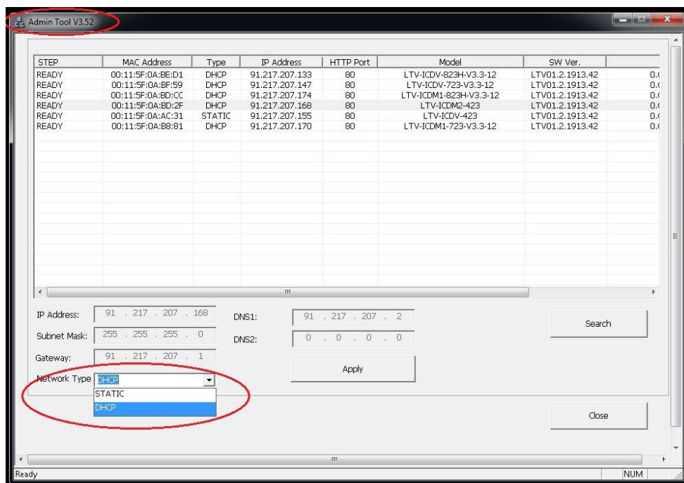
Рис.5.1. Панель Admin Tool
