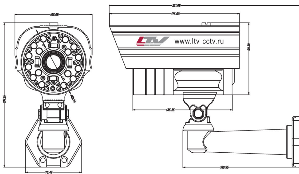
Рис.1.3.2. Габаритные размеры видеокамеры LTV-CDH-620LH-V6-50
