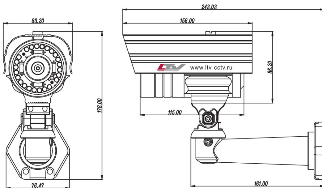
Рис.1.3.1. Габаритные размеры видеокамеры LTV-CDH-620LH-V2.8-12
