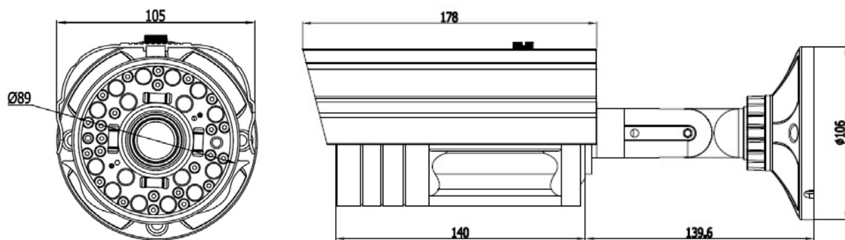
Рис.1.3.2. Габаритные размеры видеокамеры LTV-CDH-621LH-V6-50
