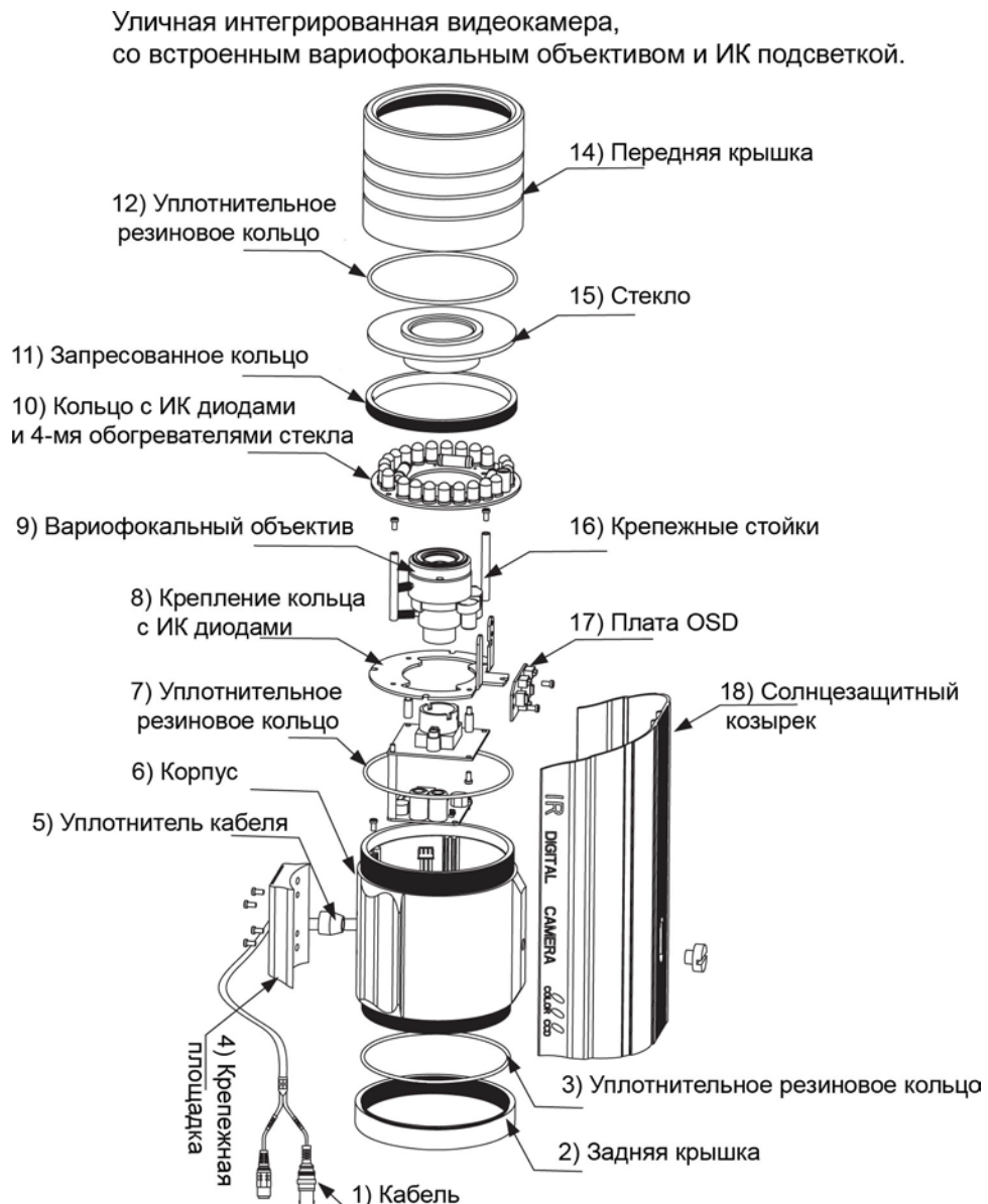
Рис.2.1 Описание видеокамеры LTV-CDH-620(1)LH-V
