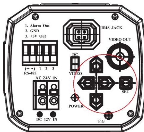
Рис.4.2.1. Управление OSD-меню видеокамеры LTV-CDH-421W
