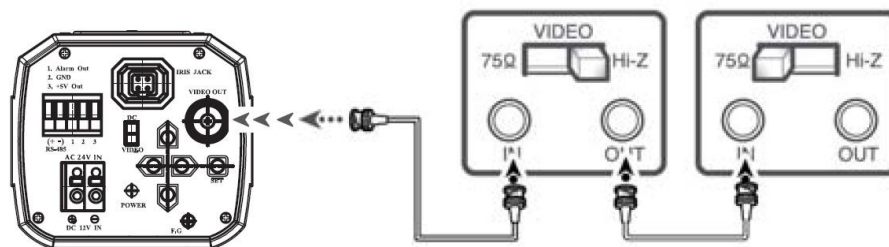
Рис.3.1.2. Подключение видеокамеры LTV-CDH-421W к монитору
