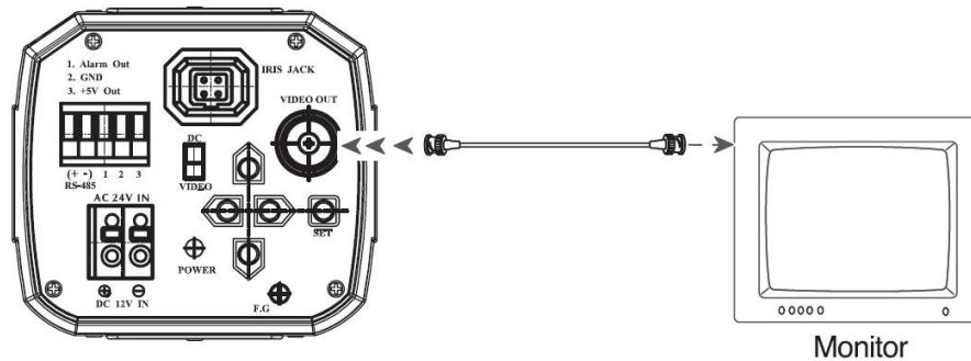
Рис.3.1.1. Подключение видеокамеры LTV-CDH-421W к монитору
