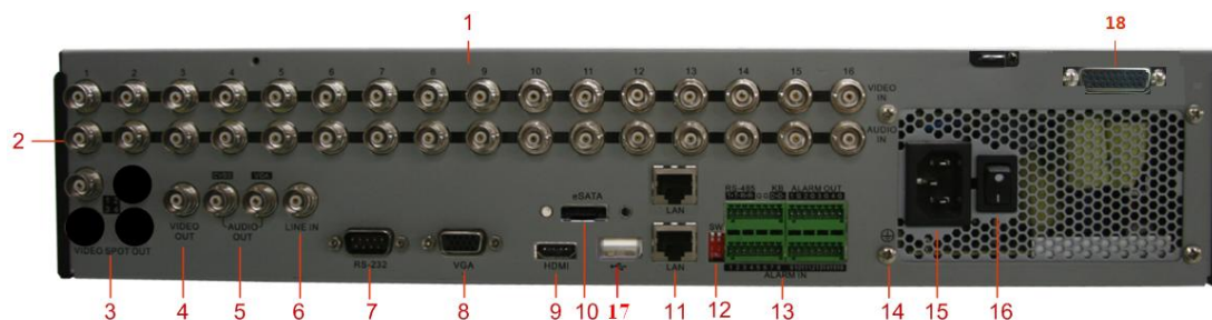
Рис.1.4. Задняя панель
