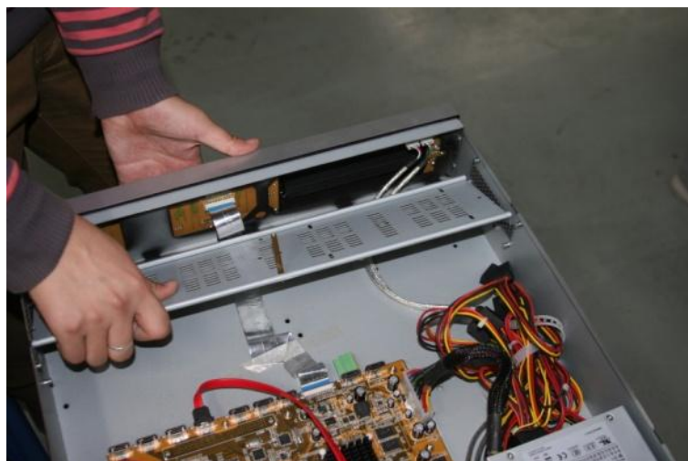
Рис.1.10. Монтаж пластины для установки дополнительных HDD
