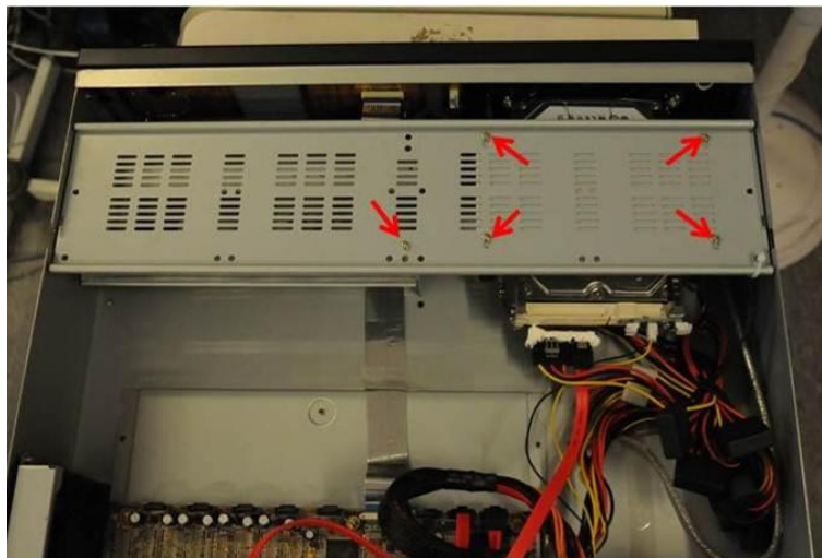
Рис.1.6. Болты на верхней пластине
