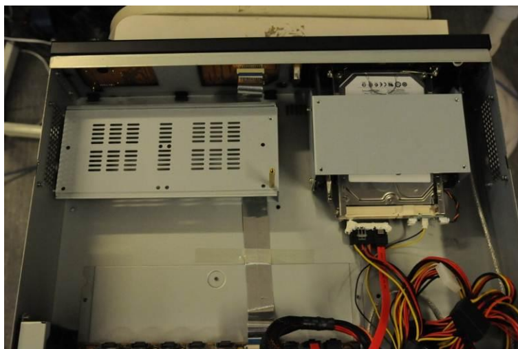
Рис.1.7. Снятие верхней пластины
