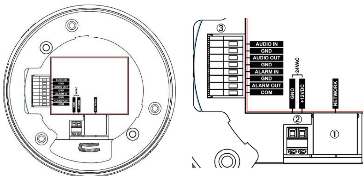
Рис.2.1.1. Задняя панель видеоканеры LTV-ICD*-723(L)-V3-9
