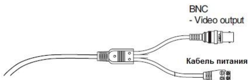
Рис.3.2.1. Подключение питания видеокамеры LTV-CDH-621L(40)HW-V
