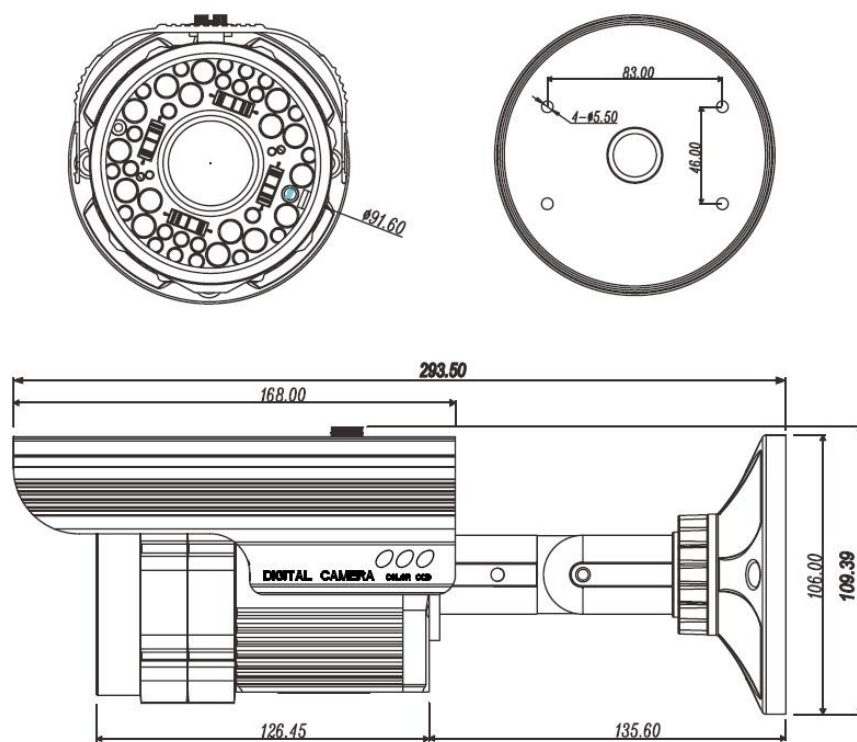
Рис.1.3.3. Габариты LTV-CDH-621L40HW-V5-50
