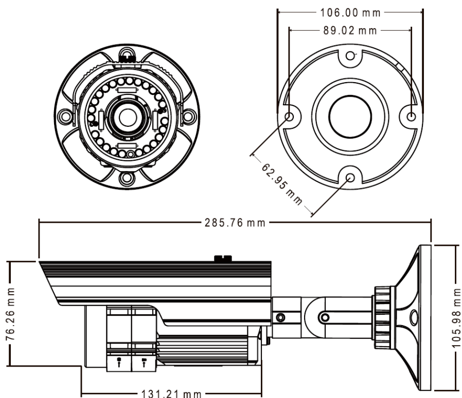
Рис.1.3.2. Габариты LTV-CDH-621LHW-V5-50
