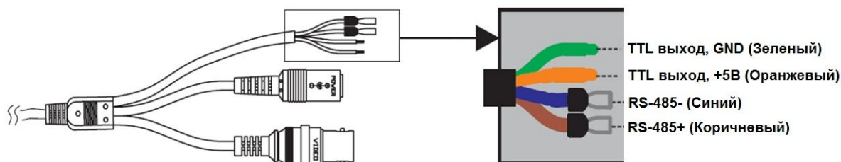
Рис.3.3.1. Подключение интерфейса RS-485 и тревожного выхода видеокамеры LTV-CDH-621L(40)HW-V
