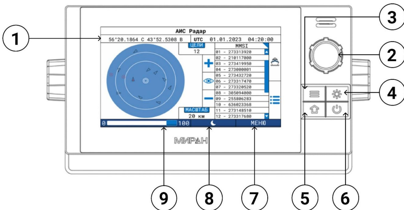
Рисунок 2 - Лицевая панель устройства
