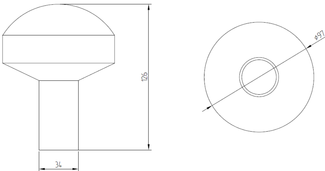
Установочные размеры блока отображения информации «ДИ-7» для установки устройства в пульт
