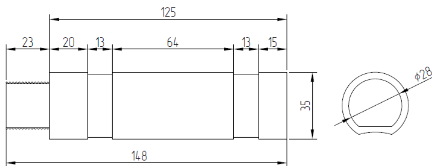
Габаритные размеры антенны «ГНСС-10-2»
