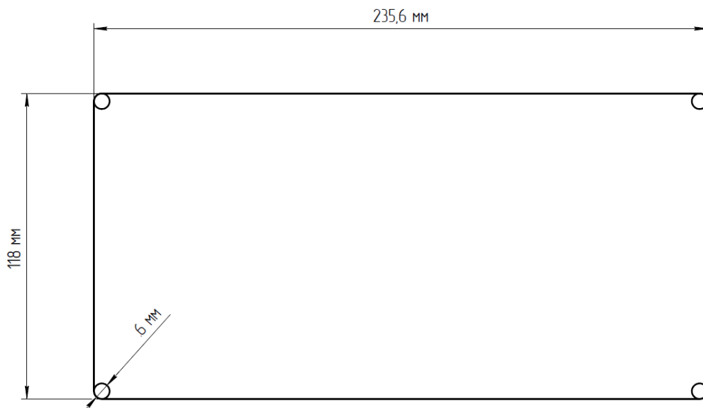
Установочные размеры блока отображения информации «ДИ-7» для установки устройства в пульт
