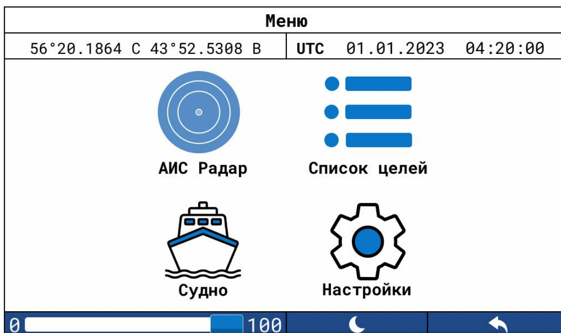
Рисунок 6 – Окно «Меню»
