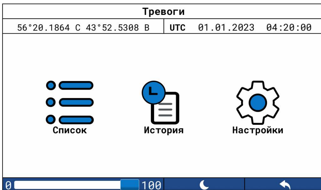
Рисунок 19 – Окно «Тревоги»
