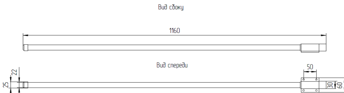
Габаритные размеры антенны УКВ
