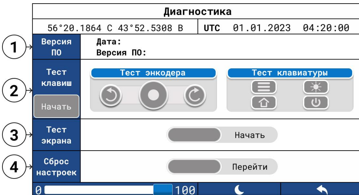
Рисунок 27 – Окно «Диагностика»
