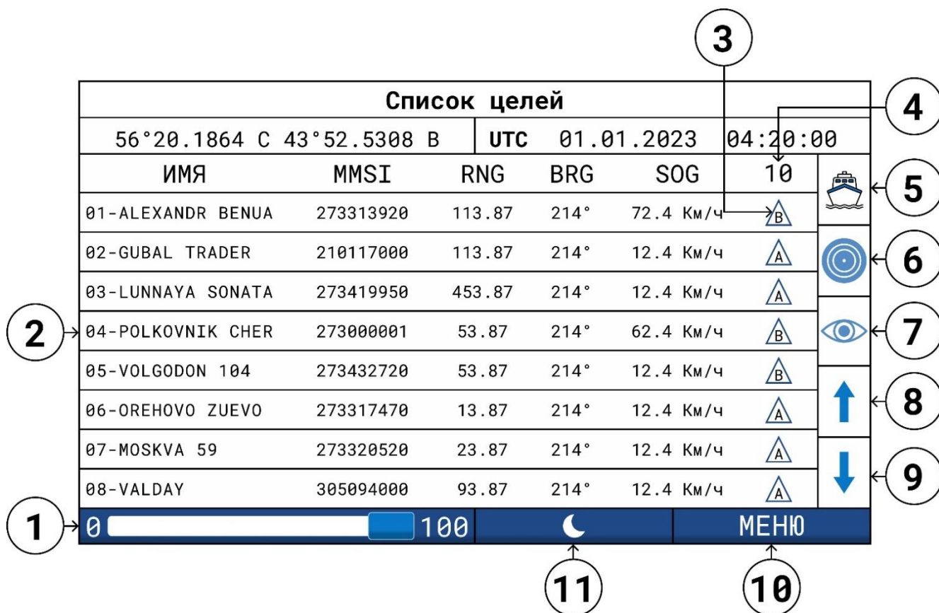
Рисунок 10 - Список целей
