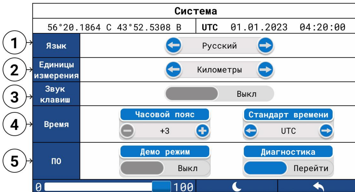
Рисунок 26 – Окно «Система»
