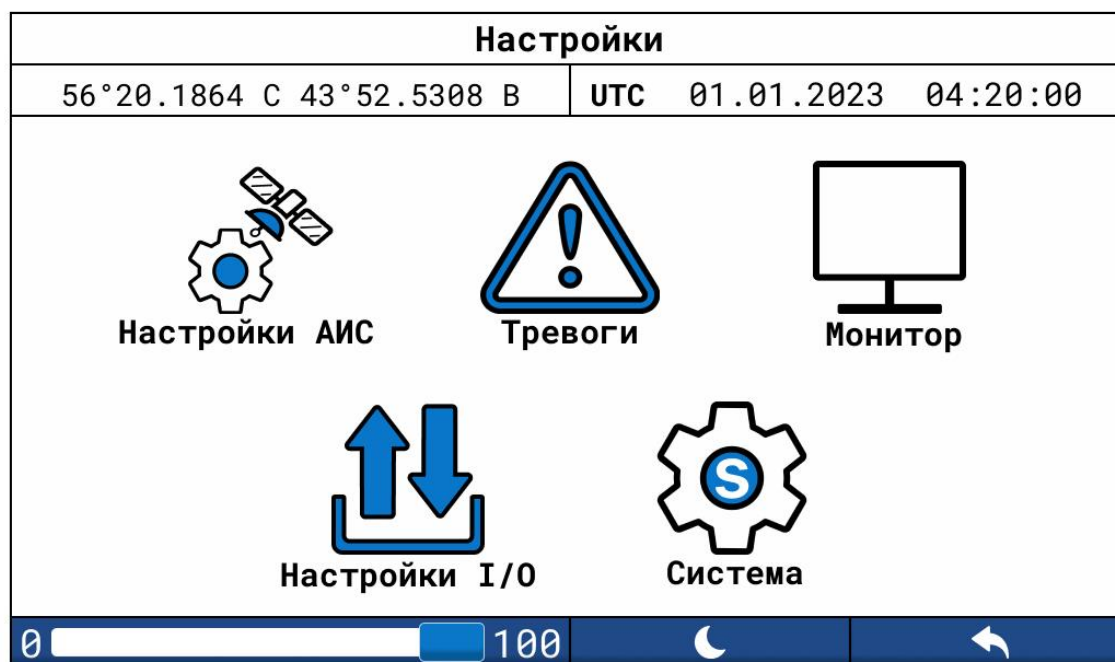
Рисунок 16 – Окно «Настройки»
