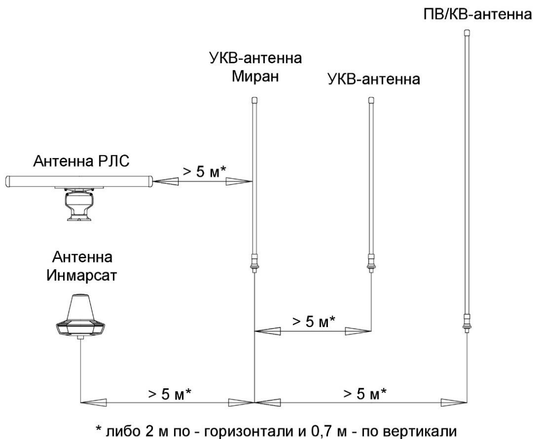
Установка антенн
