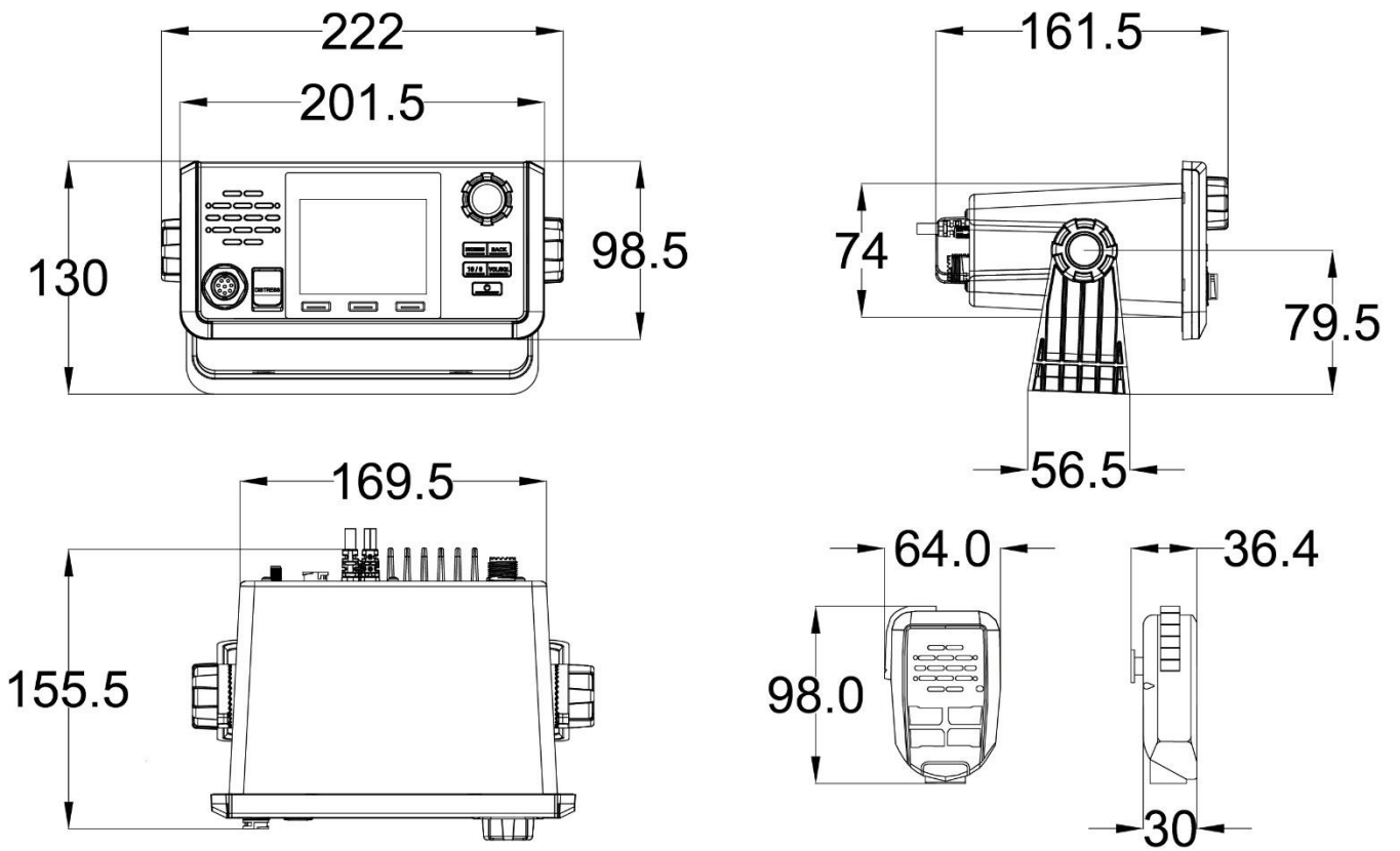
Габаритные размеры УКВ-радиоустановки с ЦИВ МИРАН «УКВ-С-1А»
