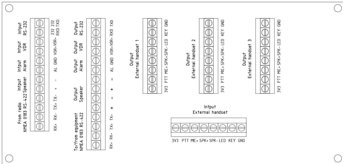
Подключение коробки соединительной «KC01»
