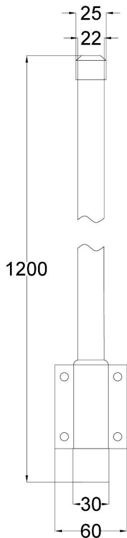
Габаритные размеры УКВ-антенны «АШ-1,2-01»
