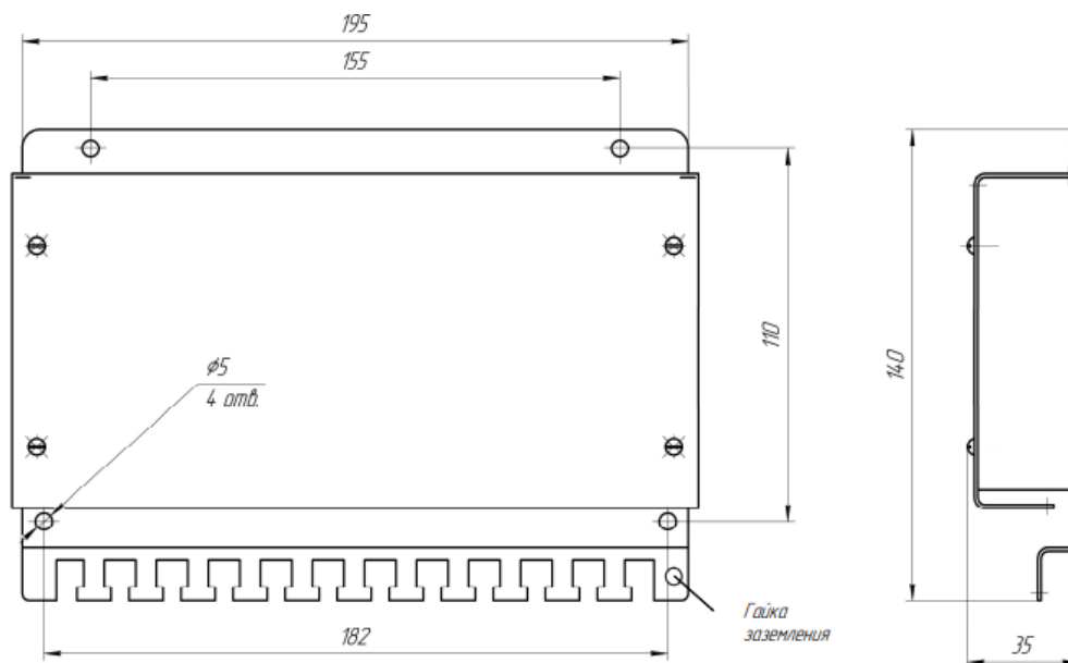
Габаритные размеры УКВ-антенны «АШ-1,2-01»
