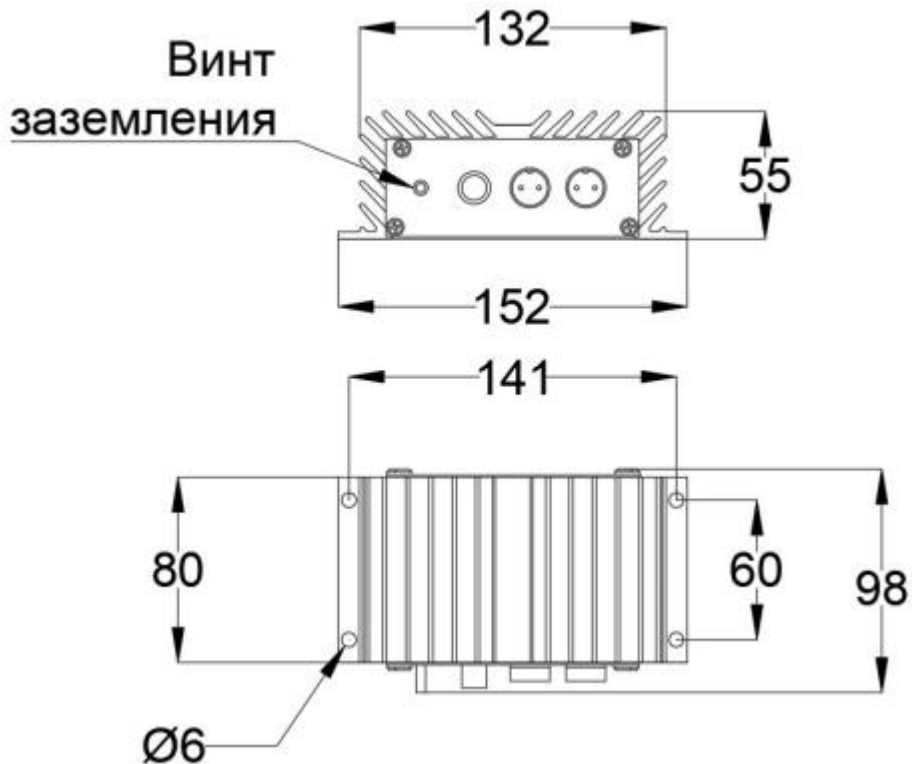
Габаритные размеры преобразователя напряжения «ПН24/12-20»
