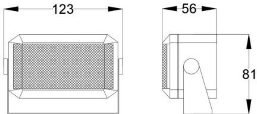
Габаритные размеры громкоговорителя «5ГП»
