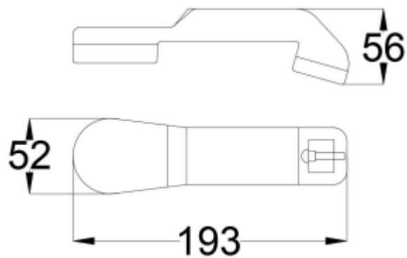
Габаритные размеры громкоговорителя «ТУ-ПВ-1А»
