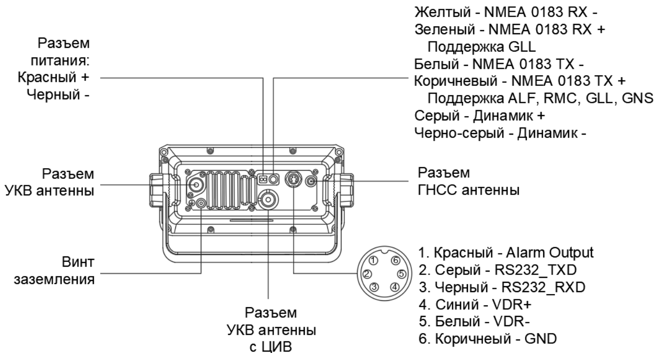
Подключение УКВ-радиостановки с ЦИВ МИРАН «УКВ-С-1А»
