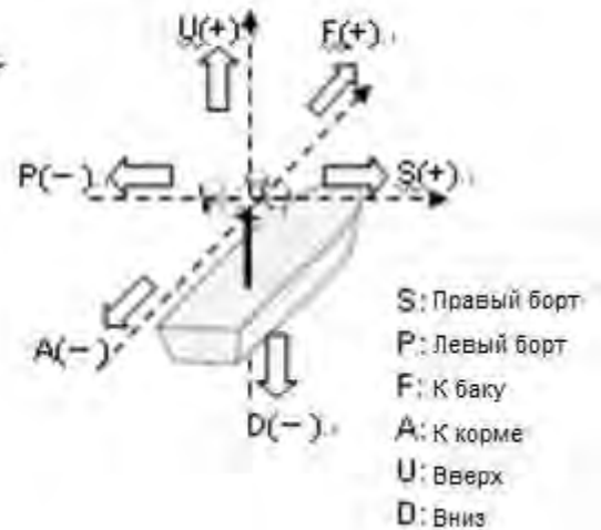
<СИСТЕМА КООРДИНАТ ДЛЯ ВВОДА СМЕЩЕНИЯ>
